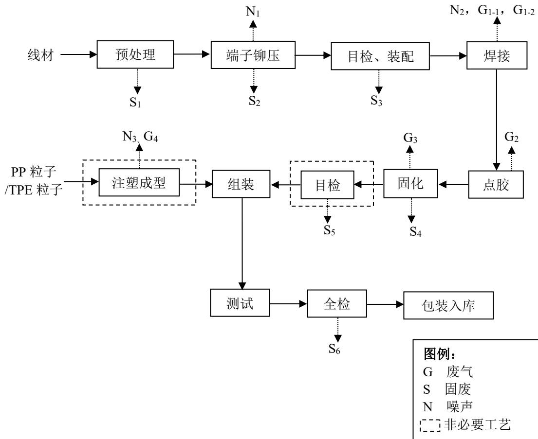
图 2-3 线束生产工艺流程图
