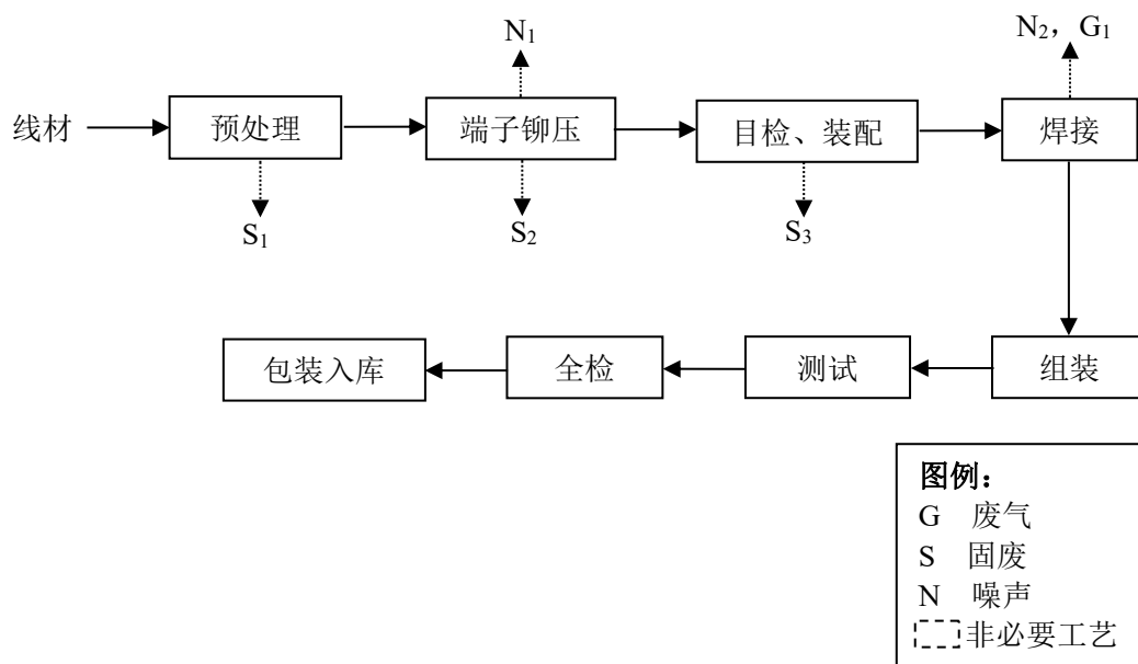
图 2-12 电池连接件工艺流程图
