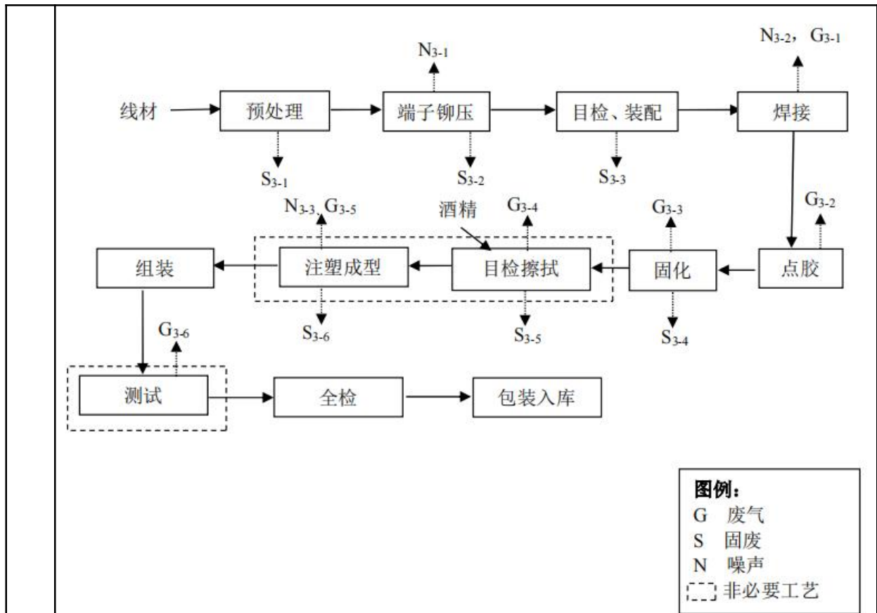
图 2-10 线束生产工艺流程图
