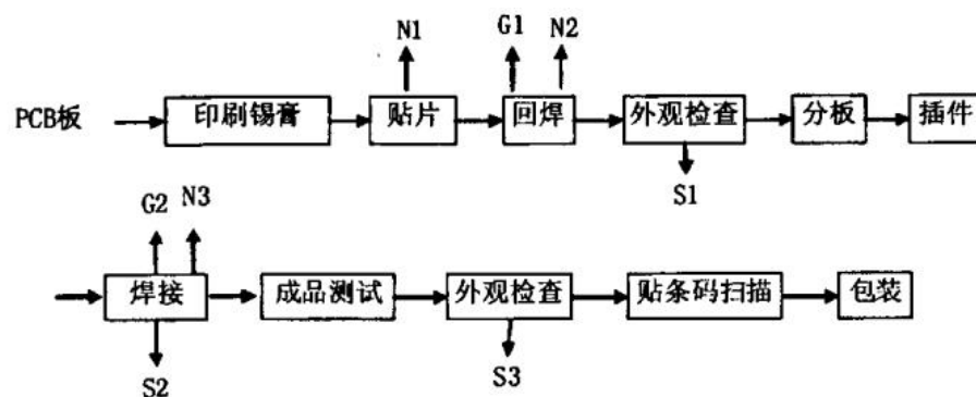
图 2-4 光电显示测试系统、新能源电池管理系统生产工艺流程图
