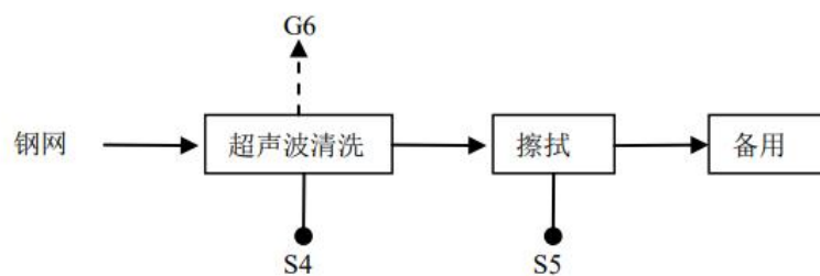
图 2-7 钢网清洗工艺流程图
