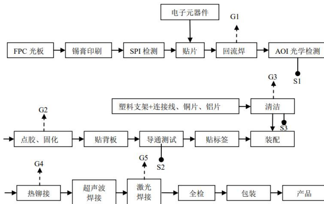
图 2-6 汽车新能源电池管理系统生产工艺流程图
